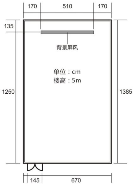
展厅平面图
