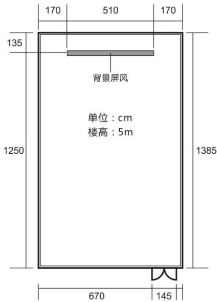
展厅平面图
