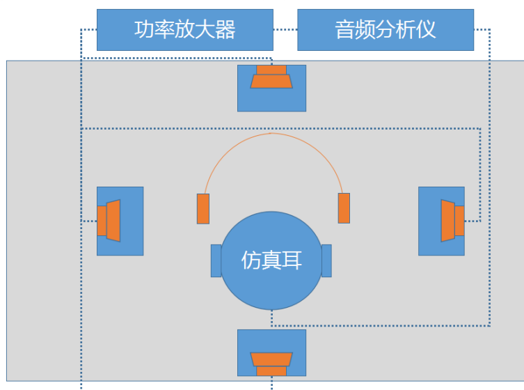
图1 测试示意图1
