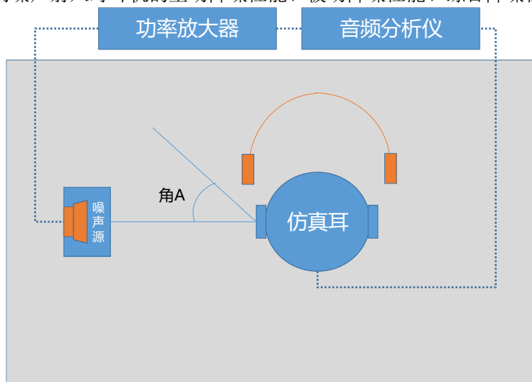
图2 测试示意图2
